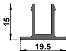
93602 kg/m 0.179
