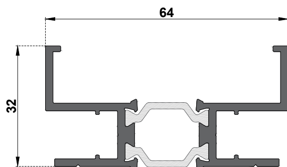
93211 kg/m 0.938
