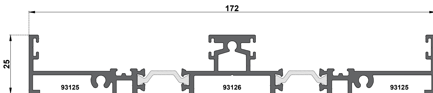
93103 kg/m 1.978
