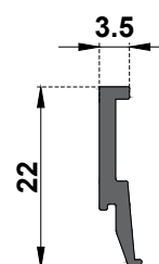
93613 kg/m 0.132
