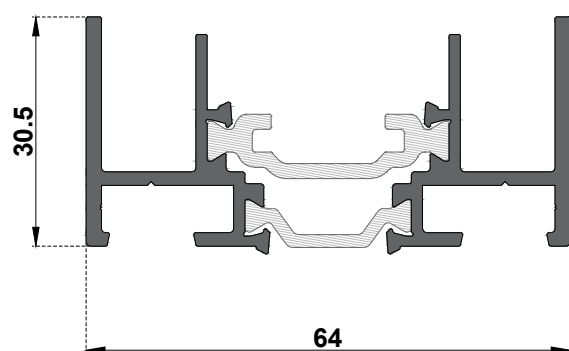
93210 kg/m 0.994
