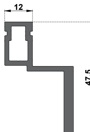
93212 kg/m 0.7
